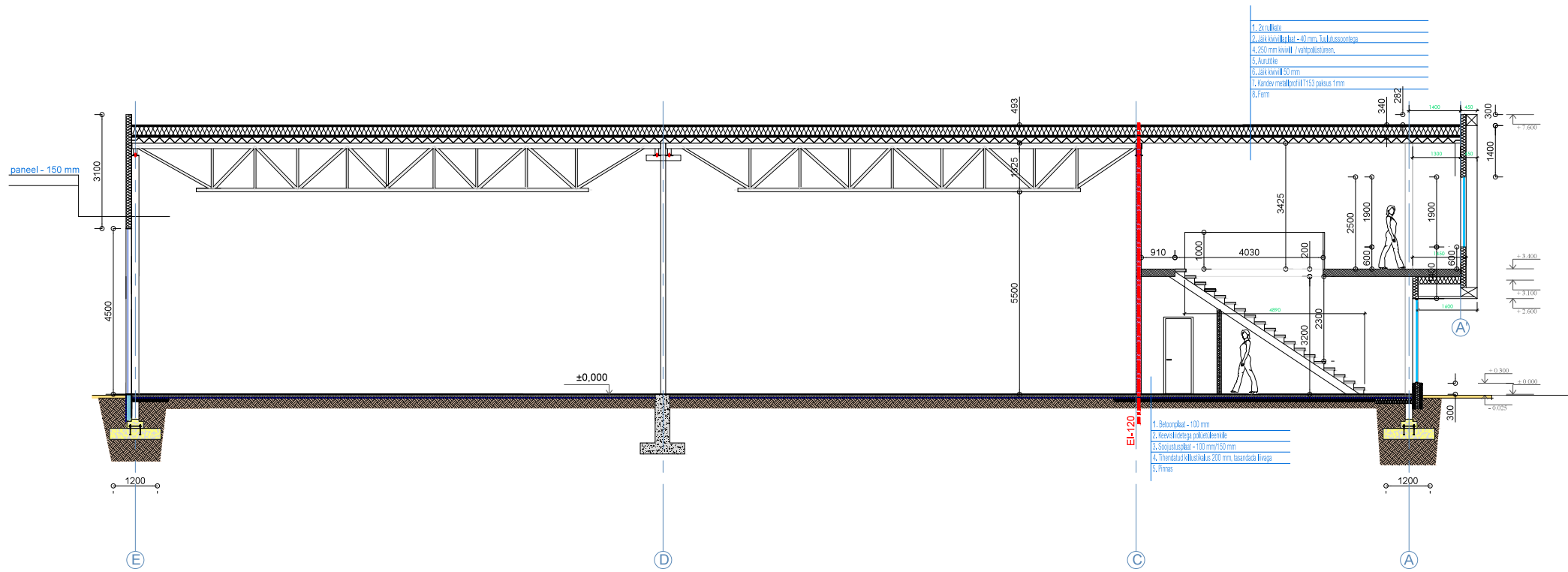
lõige A-A
